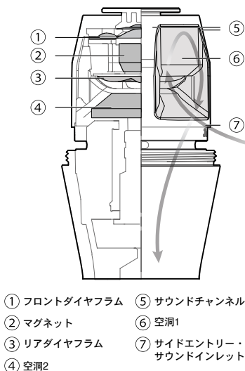
Dualdyneカートリッジ側面図
