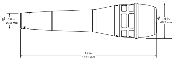
Gesamtabmessungen
