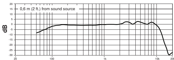
Réponse en fréquence
