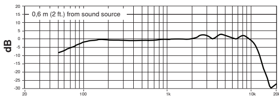
Risposta in frequenza
