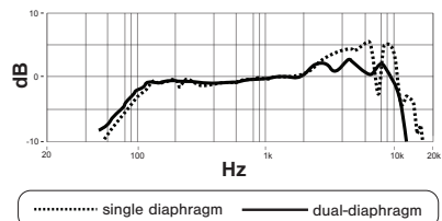
Сравнительные частотные характеристики микрофона с одной и двумя диафрагмами
