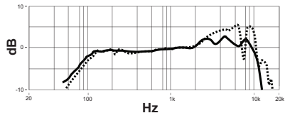
단일 다이어프램과 듀얼 다이어프램의 주파수 응답 비교
