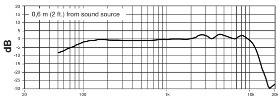
频率响应
