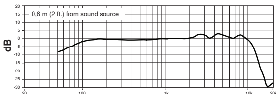
주파수 응답
