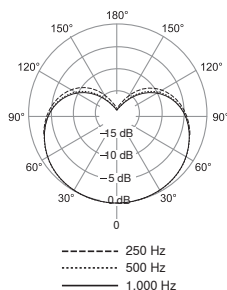
Courbe de directivité
