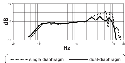
Resposta de frequência de diafragma único vs. diafragma duplo
