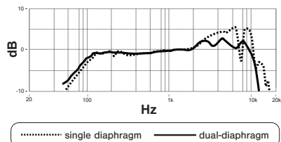
シングルダイヤフラムとデュアルダイヤフラムの周波数レスポンス
