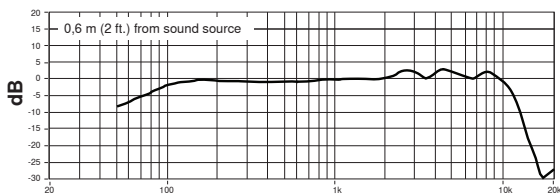
Respuesta de frecuencia
