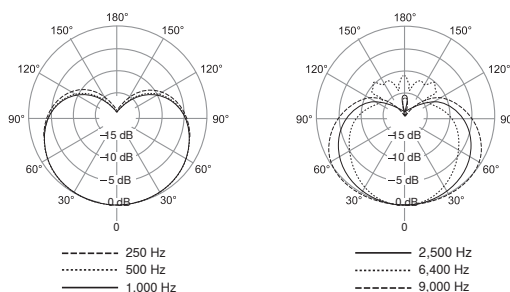
Richtcharakteristik
